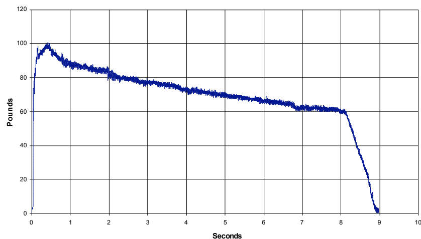
Aerotech L339W
